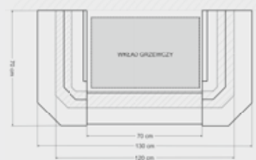
Obudowa prosta
