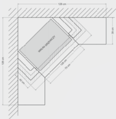
Obudowa narożna
